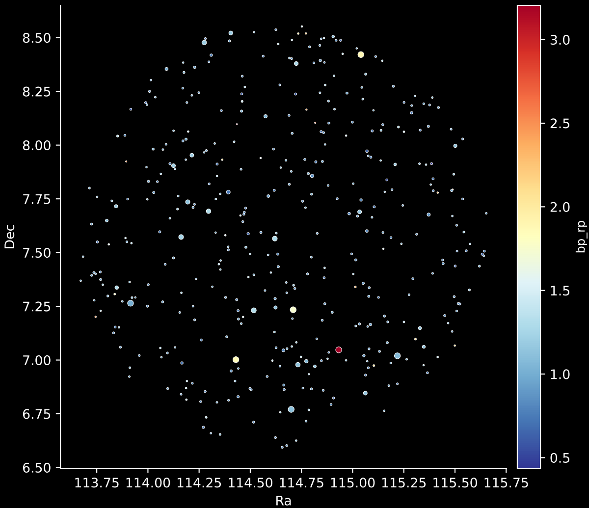
GALAH DR4 Field: [6688] Stars: 412
