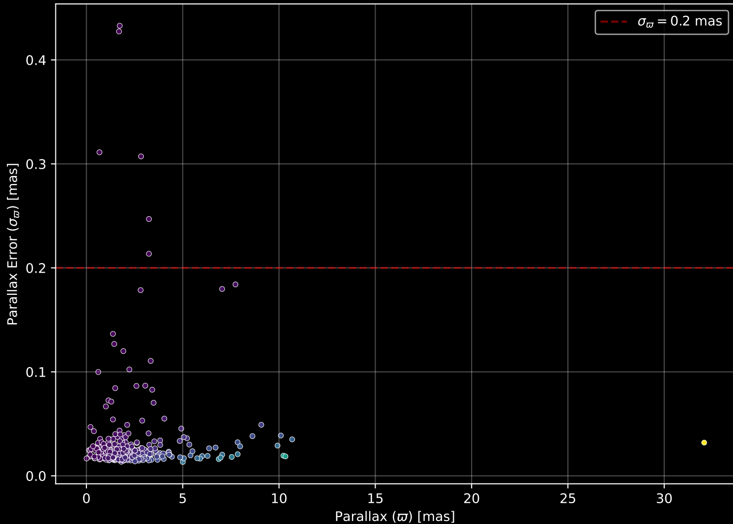
GALAH DR4 Field: [6688] Parallax Quality (n= 412)
