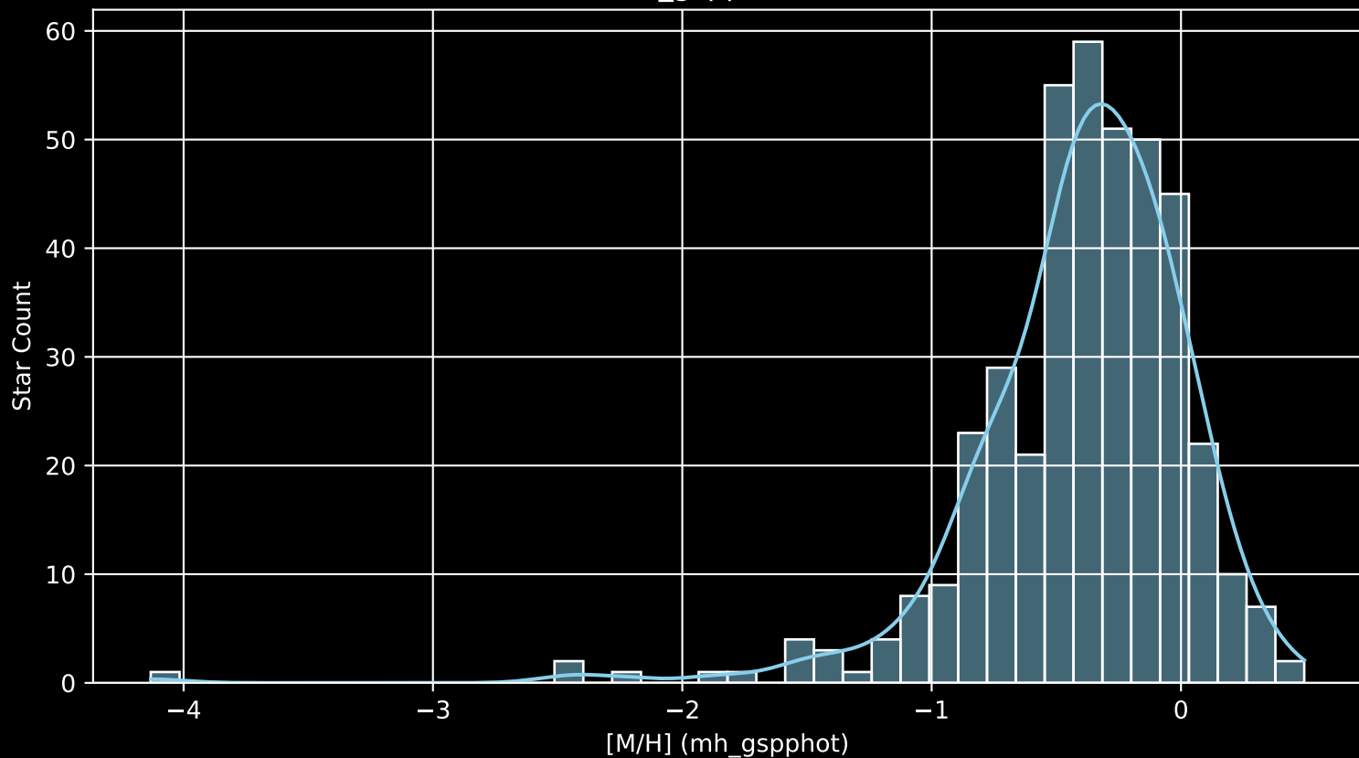
GALAH DR4 Field: [6688] [M/H] (mh_gspphot) (n= 409)
