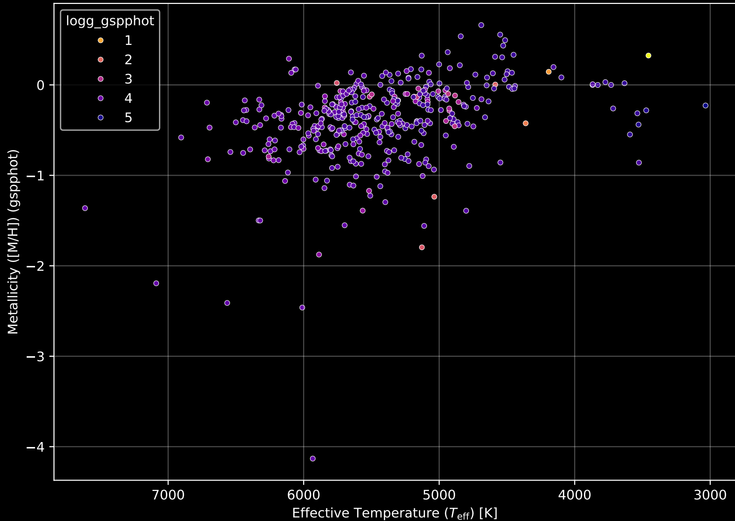
GALAH DR4 Field: [6688] Stellar Population Parameters (n= 412)
